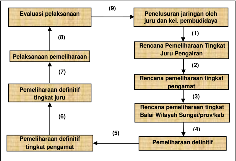
Gambar 13 - Bagan Alir Penyusunan Rencana Pemeliharaan (Sumber : Pedoman Umum Operasi dan Pemeliharaan Jaringan Reklamasi Rawa Pasang Surut)
