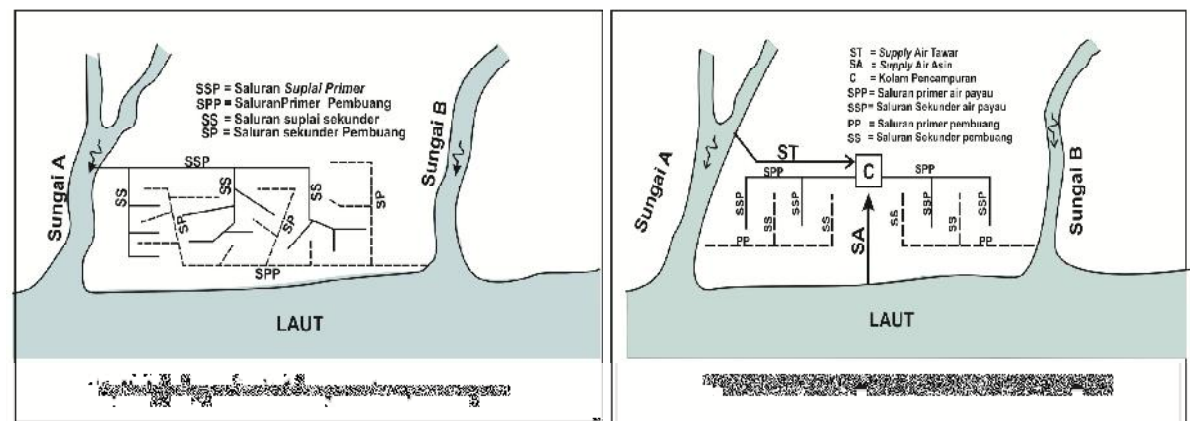
Gambar 9 - Tipe Jaringan Irigasi Tambak Dengan dan Tanpa Kolam Pencampur (Sumber : Subdit Perencanaan Teknis Direktorat Rawa dan Pantai)
