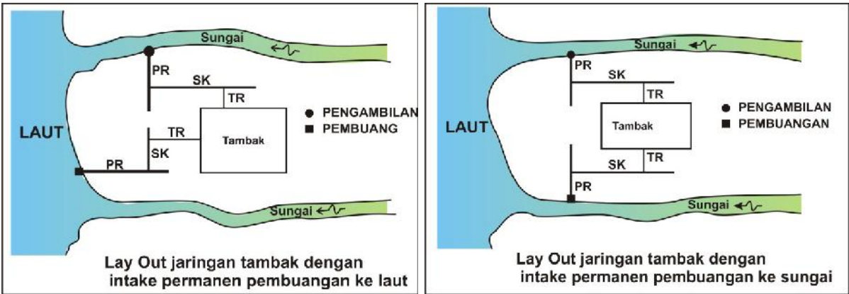
Gambar 10 - Tipe Jaringan Irigasi Tambak Dengan Bangunan Pengambil dan Pembuang Permanen (Sumber : Subdit Perencanaan Teknis Direktorat Rawa dan Pantai)
