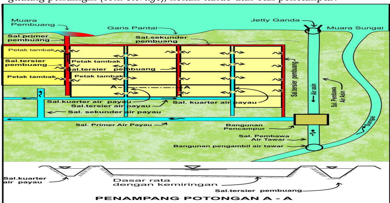
Gambar 8 - Tipe Jaringan Irigasi Teknis Tambak
